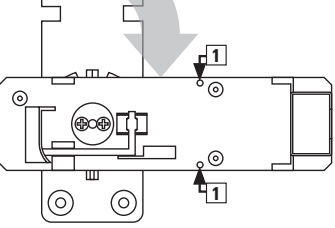
Durch Schwenken rastet der Türwächter ein und gibt den Betätigungsweg der Klinke frei. Gleichzeitig ertönt ein Alarm.
